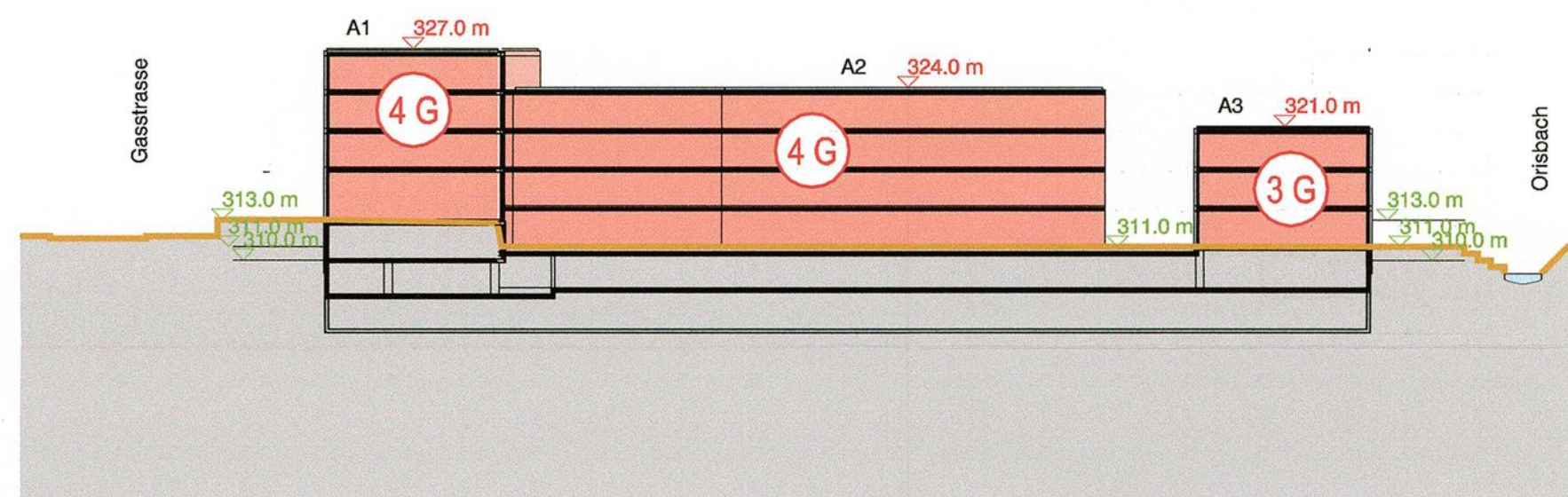
Schnitt 4-4'
