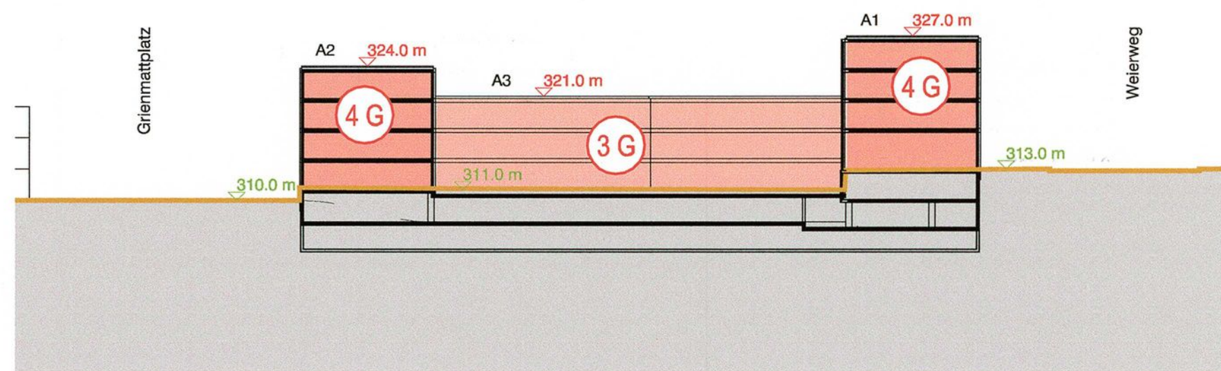
Schnitt 4-4'
