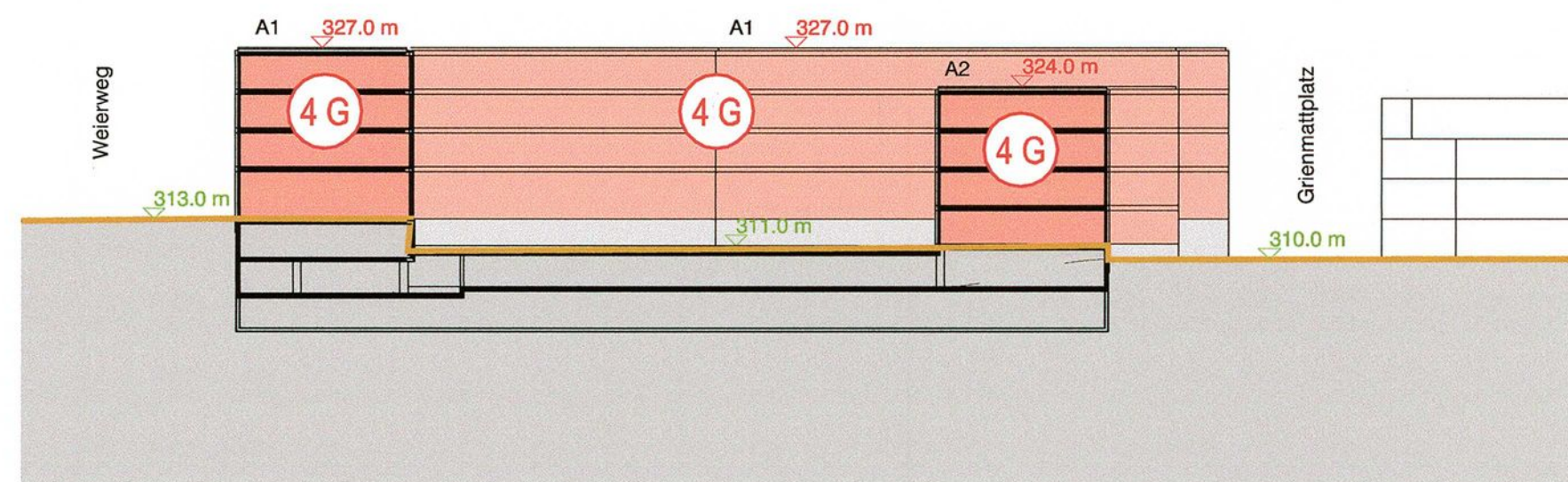
Schnitt 2-2'
