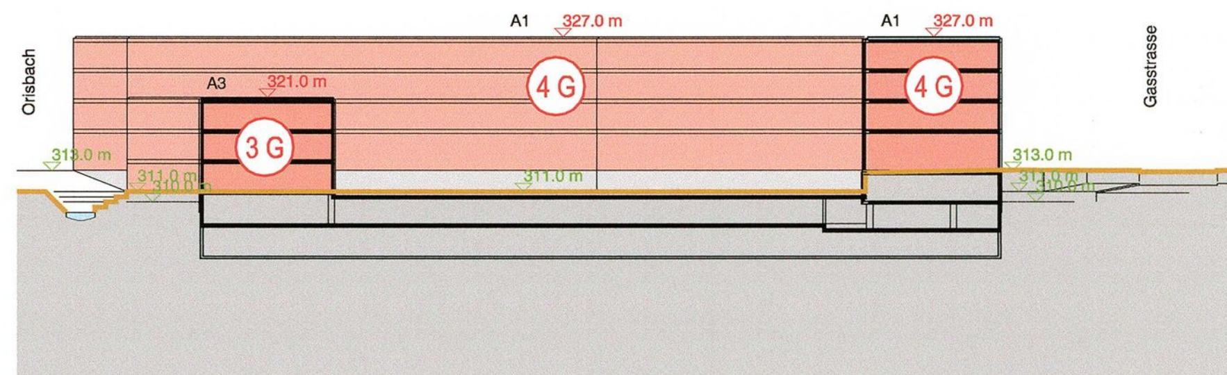
Schnitt 1-1'
