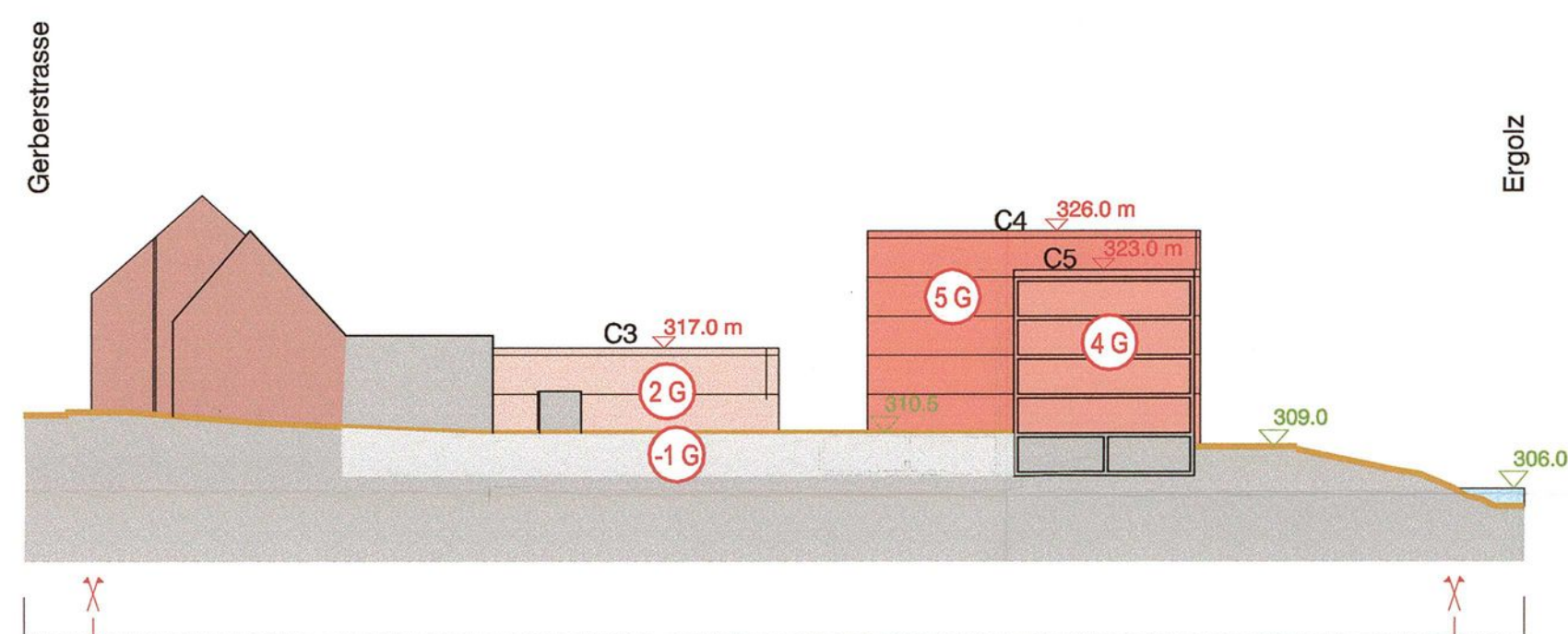
Schnitt 2-2'
