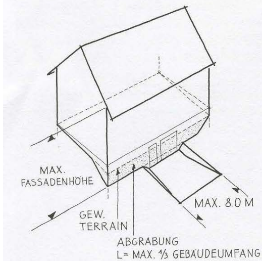
b) Abgrabungen
