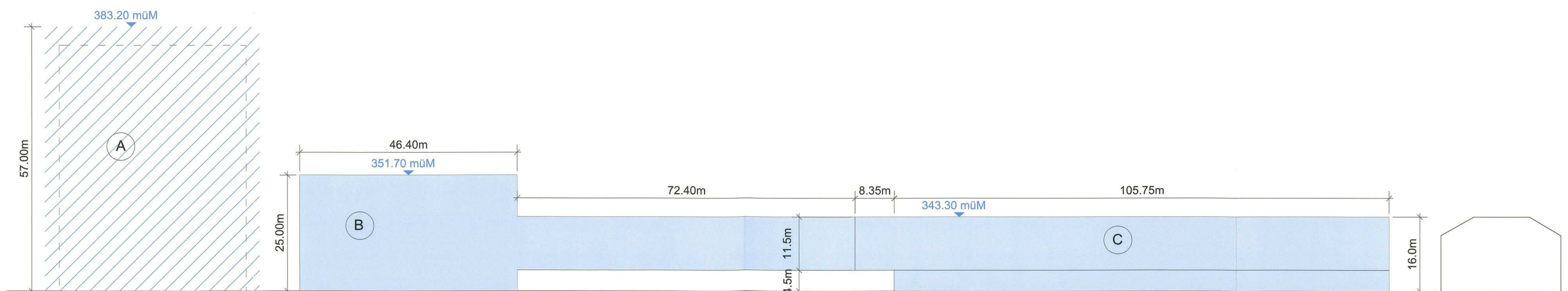
SCHNITT Masse, Dachkoten
