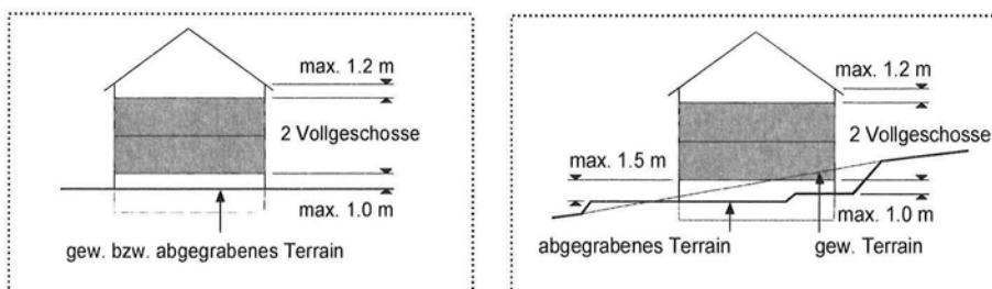
Prinzipskizze Vollgeschossezahl
