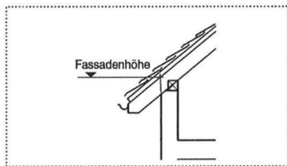
Messpunkte
