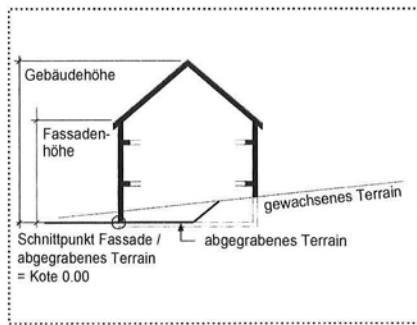
Abgrabung
