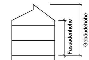
Satteldach mit einem in der Höhe versetzten First
