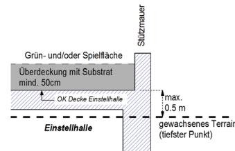
Überdeckte Einstellhalle:
