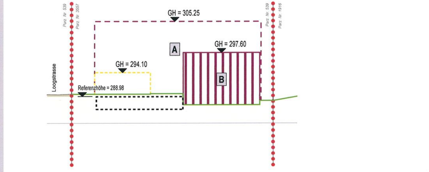
Schnitte 1 : 500
