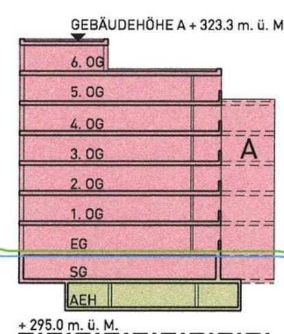
SCHNITT A-A 1:500
