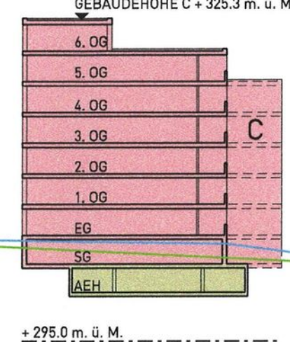
SCHNITT D-D 1:500
