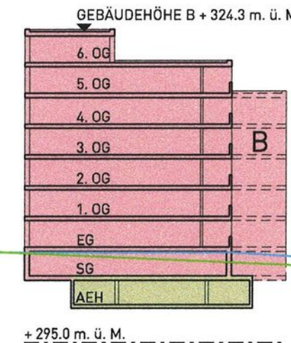
SCHNITT C-C 1:500
