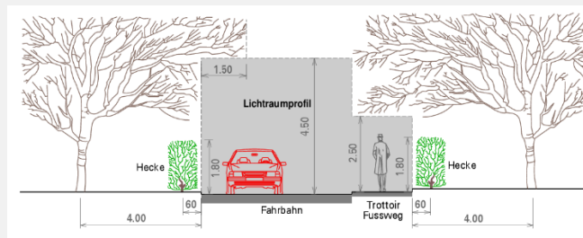
Prinzipiskizze Lichtraumprofil (Grundlage VSS-Normen)
