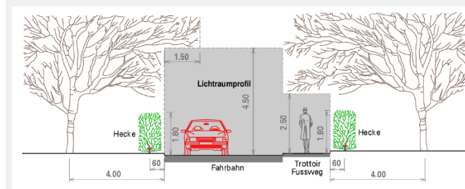
Prinzipskizze Lichtraumprofil (Grundlage VSS-Normen)
