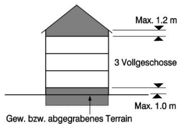
Vollgeschosszahl bei Baute in der Ebene
