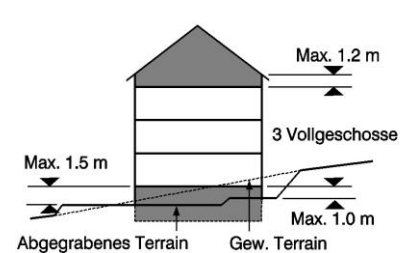
Vollgeschosszahl bei Baute im Hang
