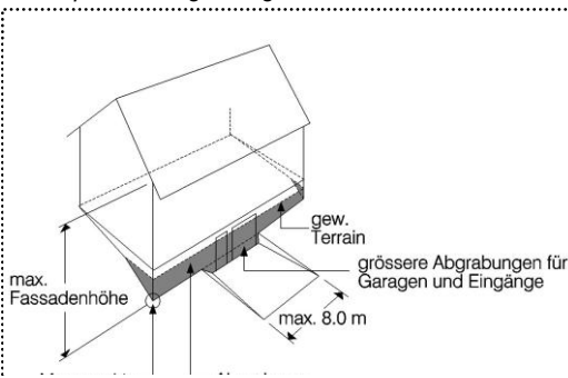
Prinzipskizze Abgrabungen am Gebäude
