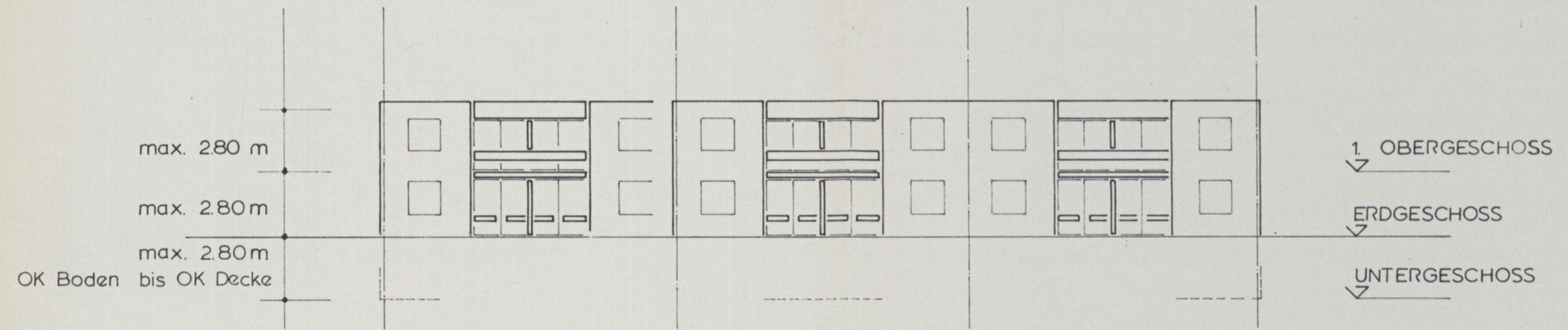
Haus 2a WEST-FASSADE
