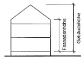
beim Satteldach
