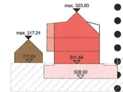
Schnitt B - B
